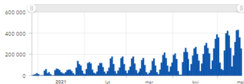
Liczba wykonanych szczepień w ujęciu dziennym
