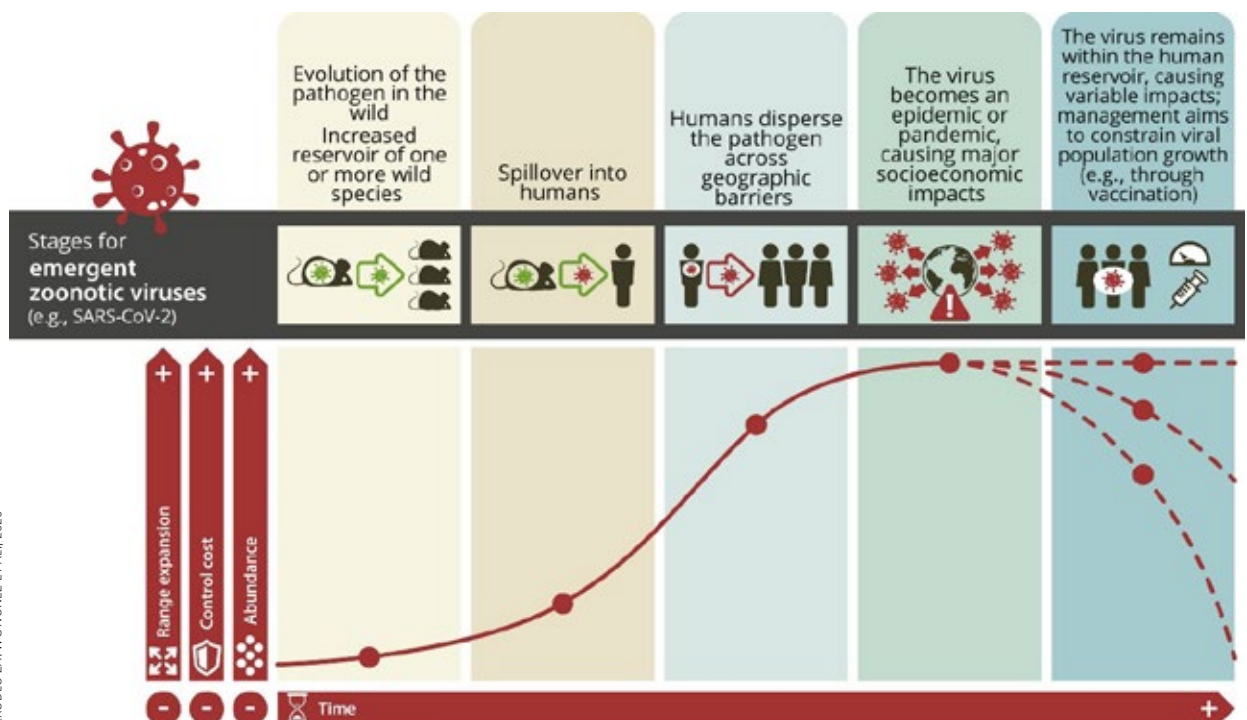
Ryc. 3 Etap rozwoju nowej epidemii
